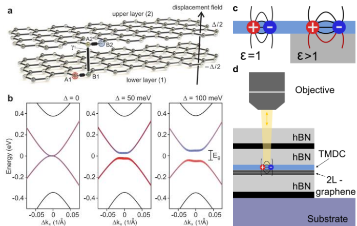
Abbildung 1: a) Kristallstruktur von Zweilagigem Graphen sowie die b) elektronische Struktur bei drei verschiedenen externen elektrischen Feldern. c) In einer Umgebung mit höherer dielektrischer Funktion werden die Coulomb-Wechselwirkungen von Exzitonen (Elektron-Loch-Paaren) in WSe_2 stärker abgeschirmt, was zu niedrigeren Bindungsenergien führt. d) Dies kann mit optischen Methoden ausgelesen werden. WSe_2 dient daher als Sensor der elektronischen Struktur in Graphen.
